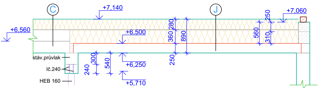
Řez 2 - 2
